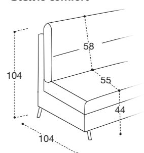
SCOCCHA POLTRONA FISSA 62
